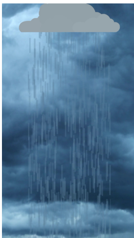
Durch höhere Temperaturen kann die Luft sieben Prozent mehr Wasserdampf aufnehmen. Das kann zu mehr Regen führen.
