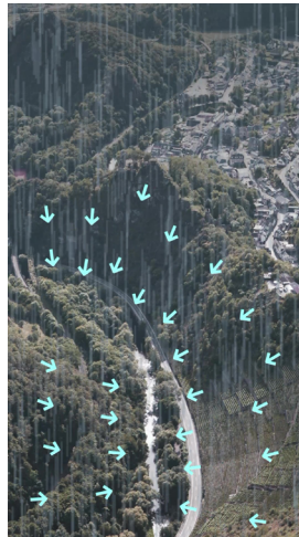
Die Ahr wurde immer breiter, schneller und höher, denn das Wasser sammelte sich in dem engen Tal.
