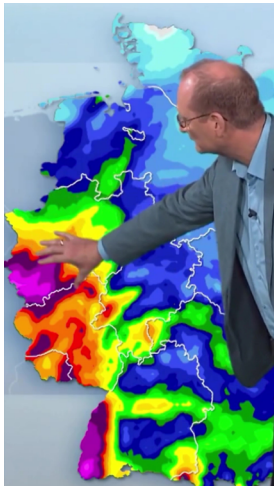
Schon Tage vor der Flut warnten die Wetterdienste vor extremen Regengüssen.
