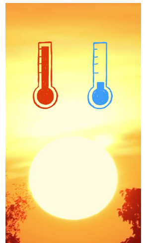
Die Gefahr für Waldbrände steigt in Zukunft. Denn heiße und trockene Sommer werden durch den Klimawandel immer häufiger.
